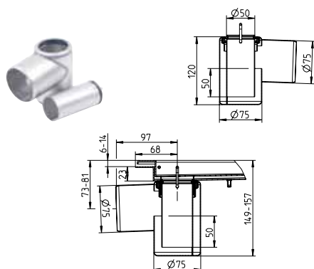
Siphonide en place
